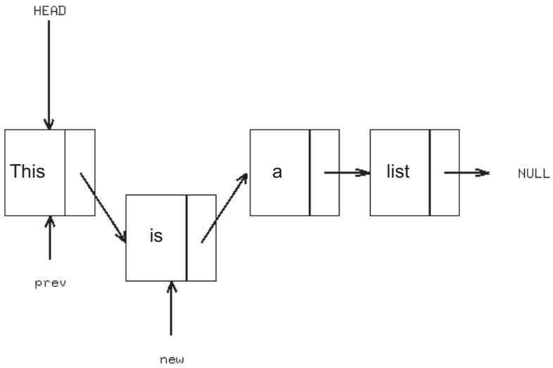
Fig. 4.10. Linked list
