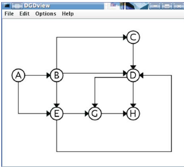
Fig. 2.11. Orthogonal layout
