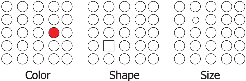
Fig. 2.4. Preattentive perception
