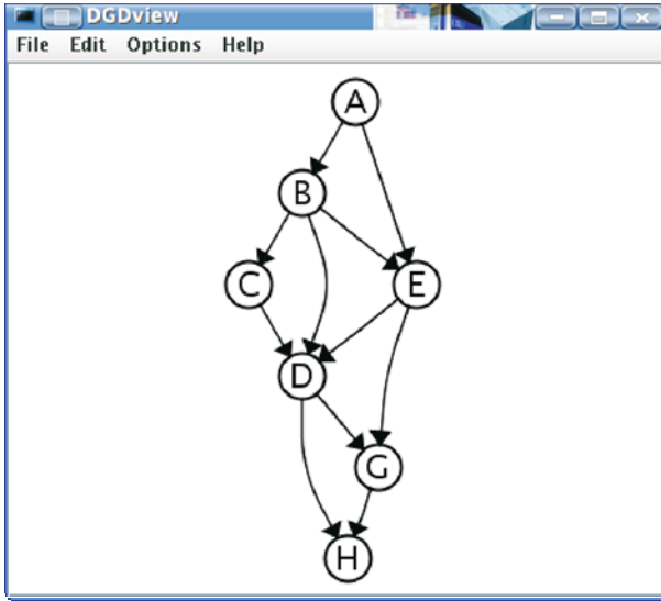
Fig. 2.10. Hierarchical layout
