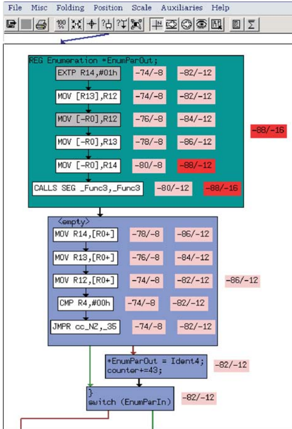
Fig. 1.4. Stack usage
